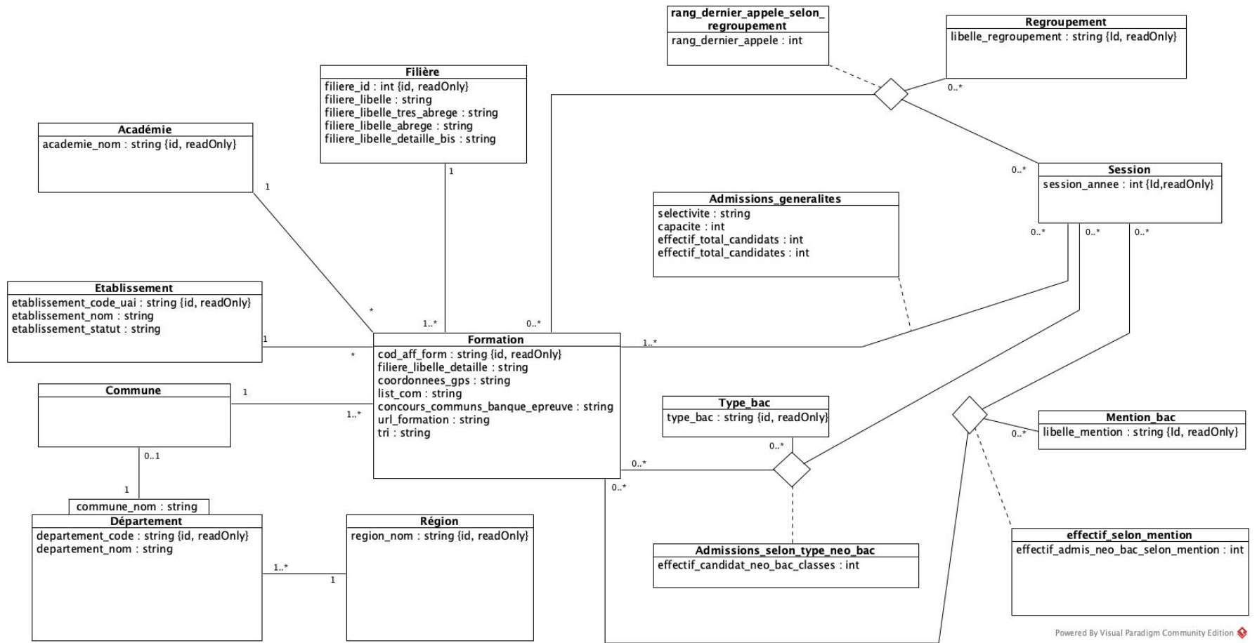
FIGURE 1 – Gestion des candidatures et des admissions dans Parcoursup - Diagramme de classe
